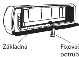
A. Vložte fixovač potrubí do slotu.
