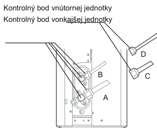
A: Nízkotlakový uzatvárací ventil B: Vysokotlakový uzatvárací ventil C & D: Vnútročné matice na rozvod
