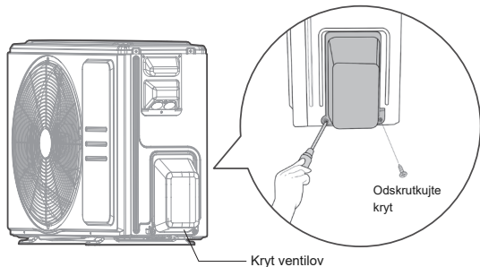
Vonkajšia jednotka
