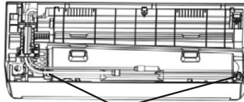
Abflussanschlüsse
